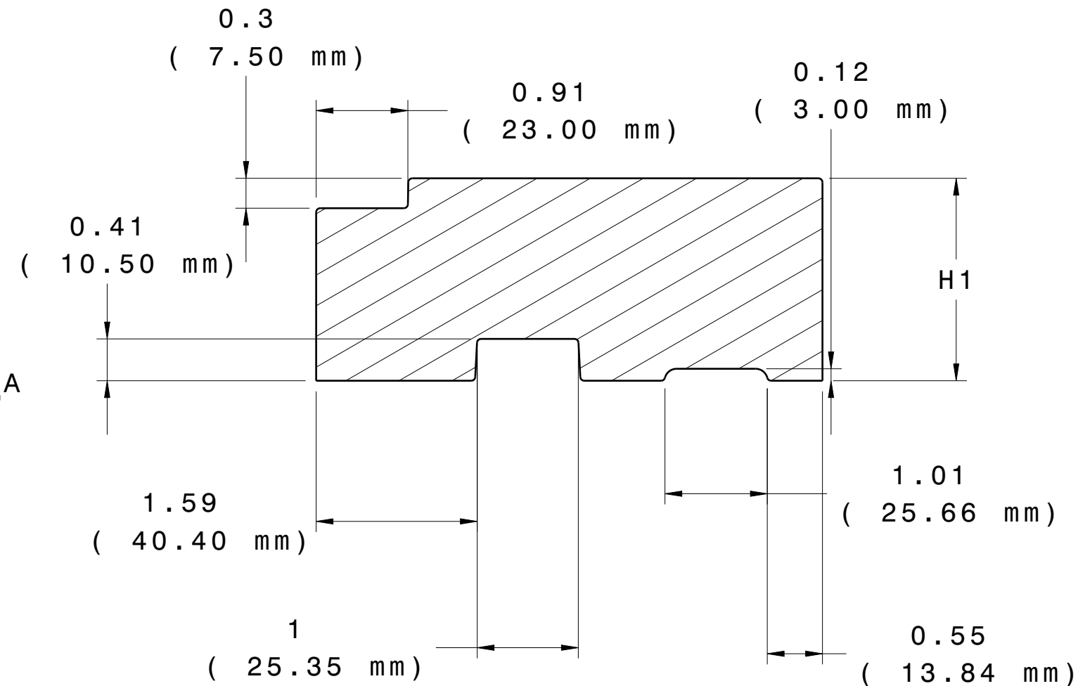
Section cut A-A Scale: 3:4
