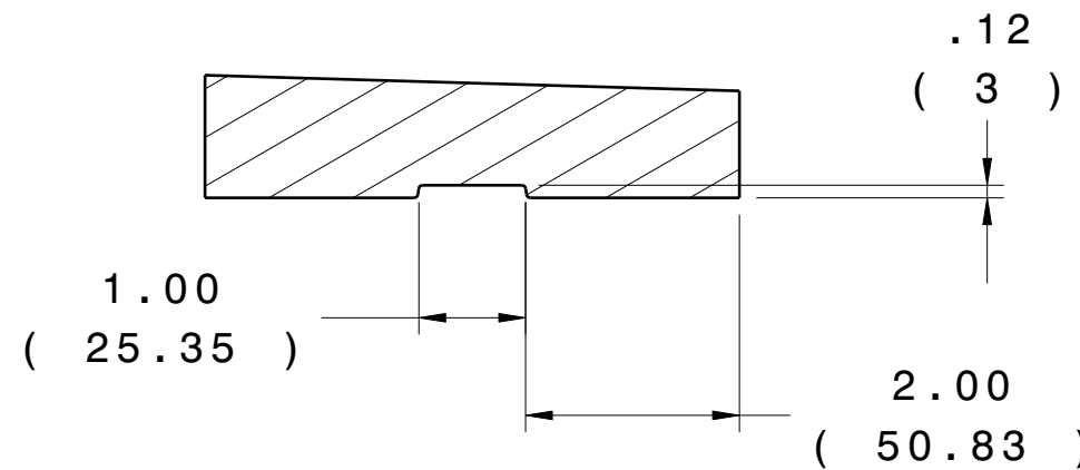
Section cut A-A Scale: 1:2
